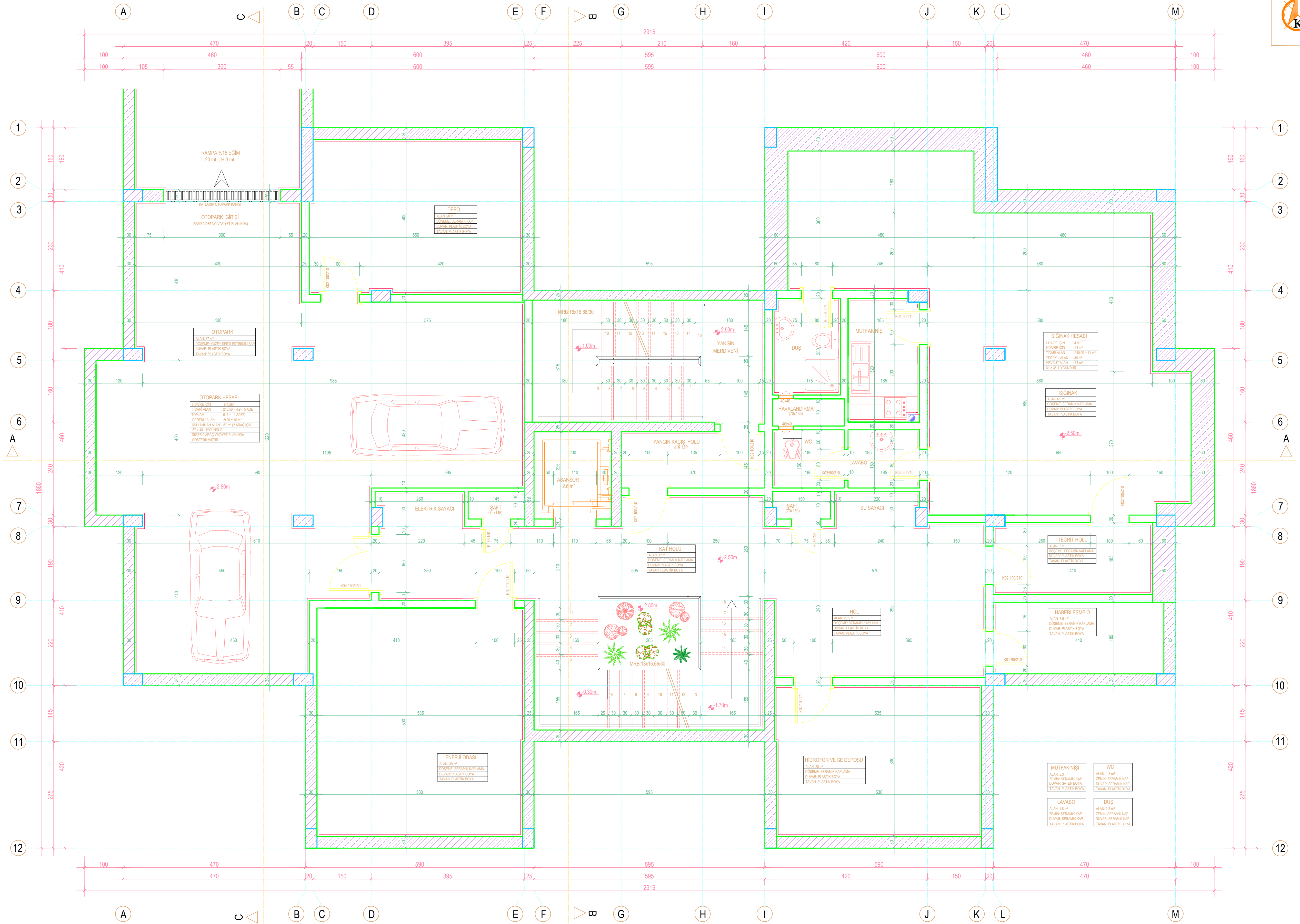
BODRUM KAT PLANI ÖLÇEK: 1/50
