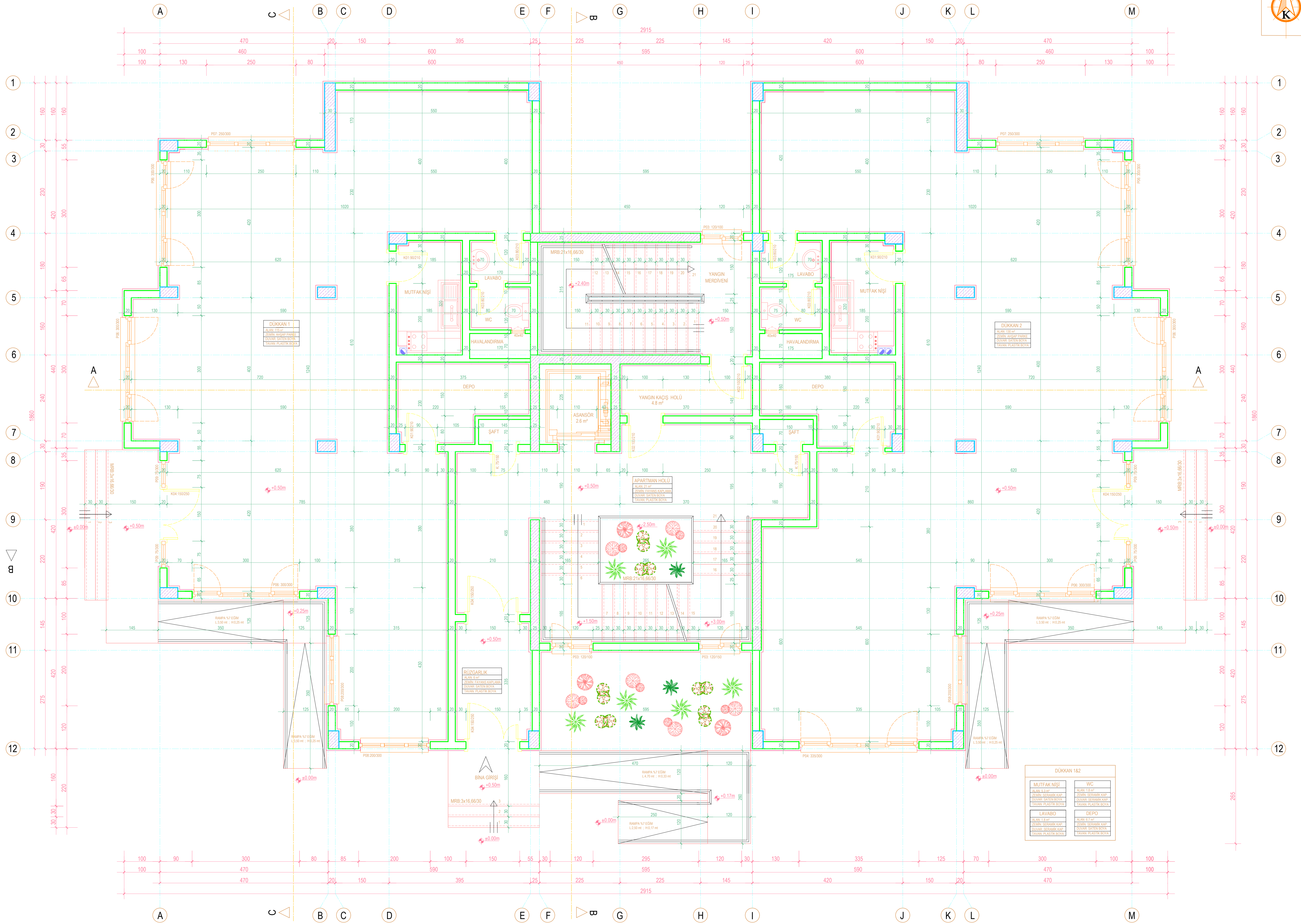
ZEMİN KAT PLANI ÖLÇEK: 1/50
