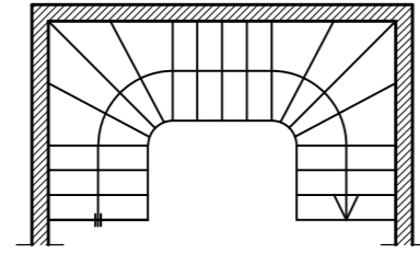
ÜÇ KOLLU ÇEYREK DÖNER MERDİVEN
