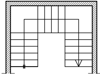
ÜÇ KOLLU KÖŞEDE SAHANLIKLI MERDİVEN
