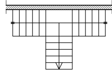
ÜÇ KOLLU ORTADA SAHANLIKLI MERDİVEN (İKİ TARAFTAN ÇIKIŞLI)
