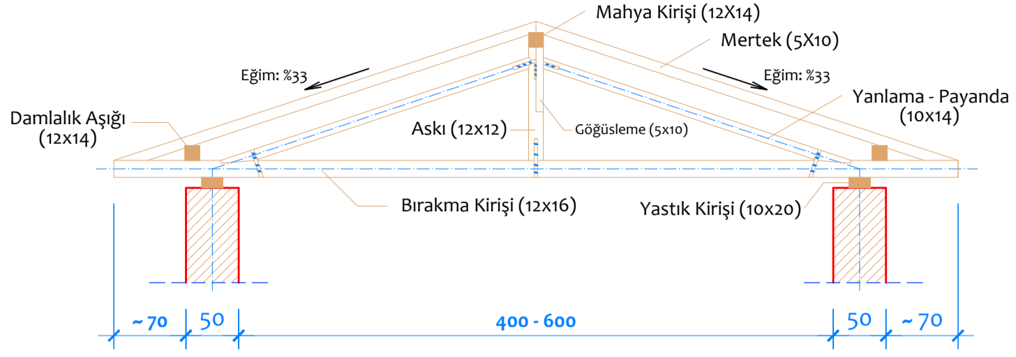
TEK ASKILI AHŞAP ASMA ÇATI MAKASI
