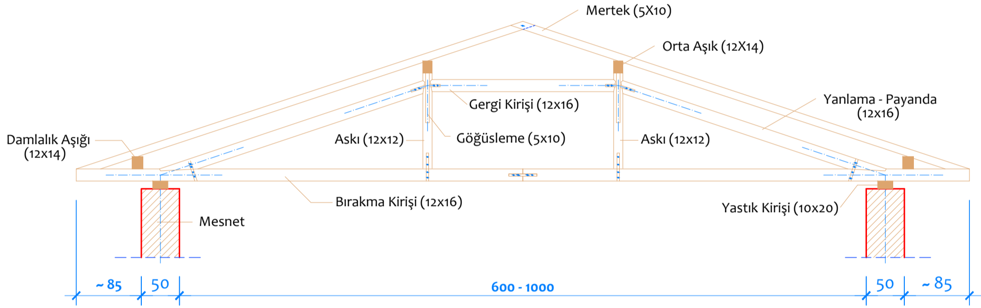
İKİ ASKILI AHŞAP ASMA ÇATI MAKASI
