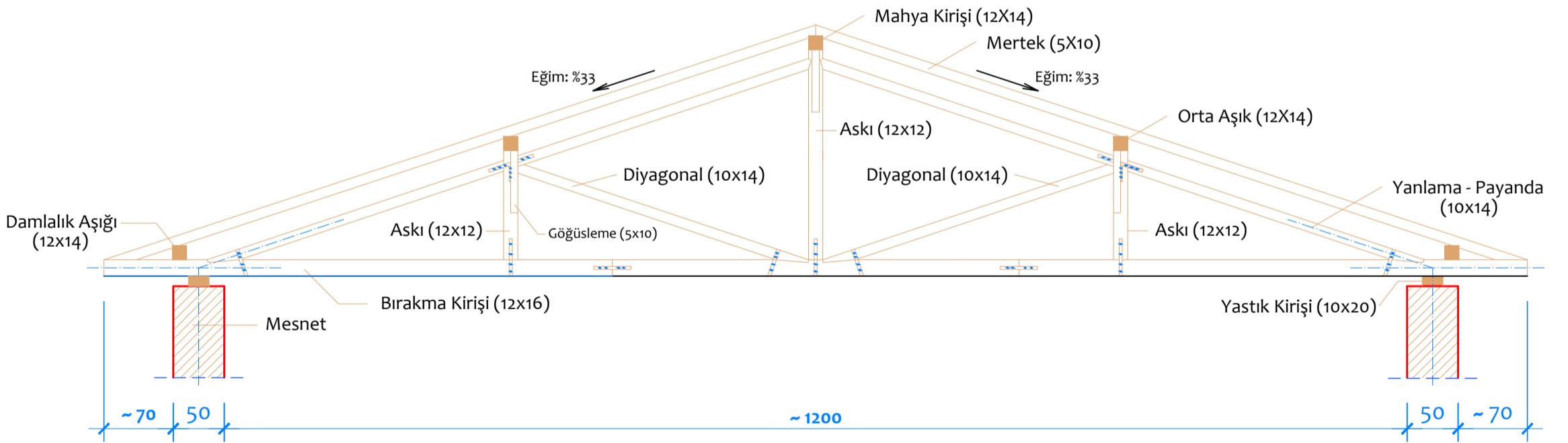
ÜÇ ASKILI AHŞAP ASMA ÇATI MAKASI
